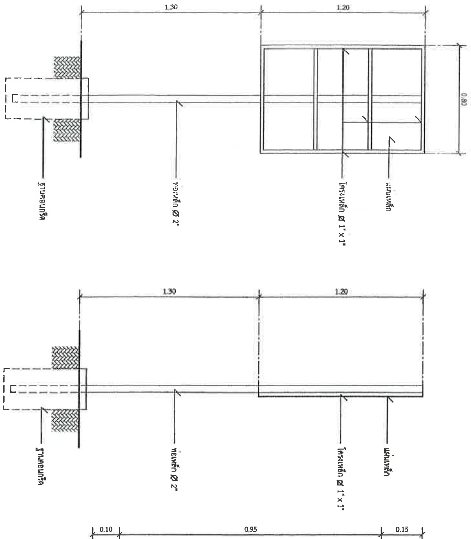
รูปด้านหลัง มาตราส่วน 1 : 20
